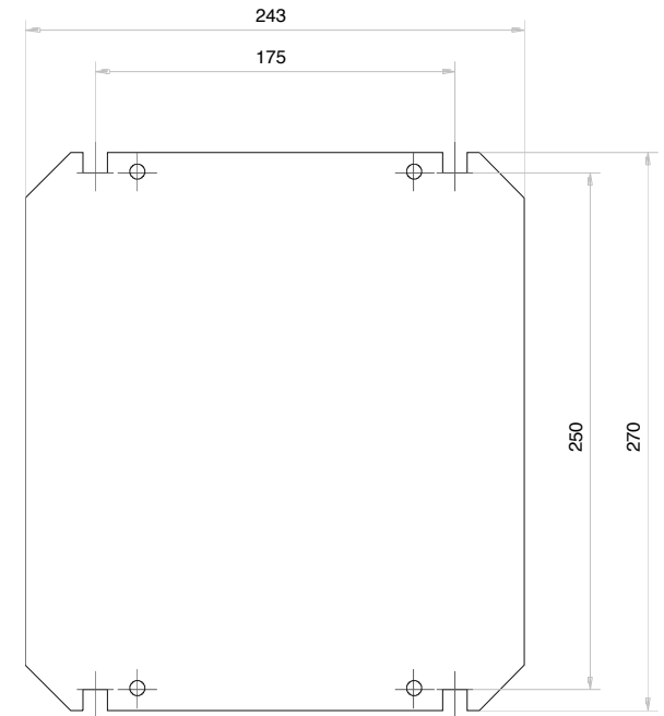
Einbauplatte sendzimirverzinkt
