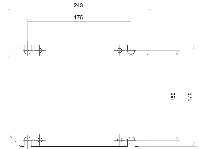
Einbauplatte sendzimirverzinkt
