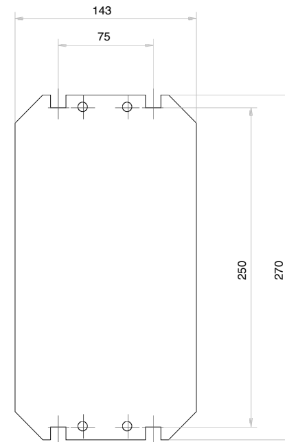
Einbauplatte sendzimerverzinkt
