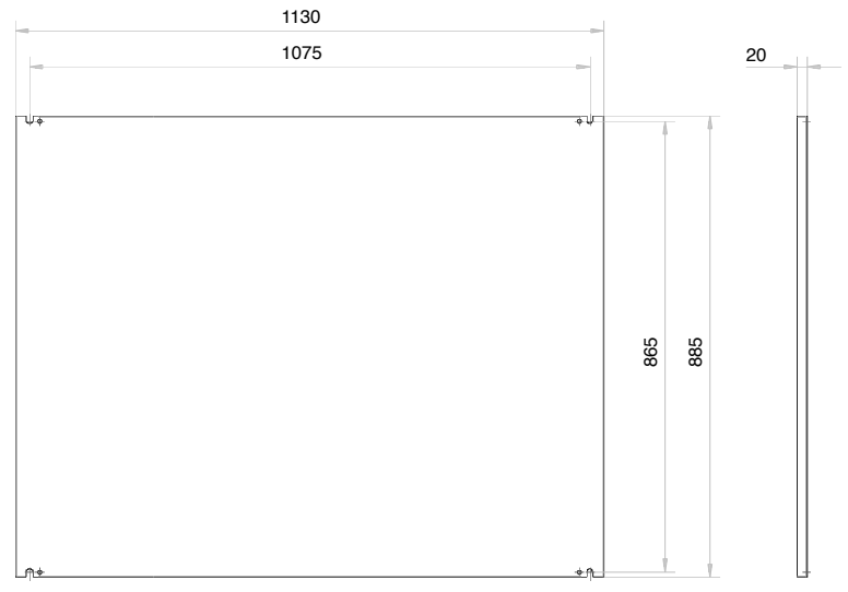
Einbauplatte sendzimirverzinkt
