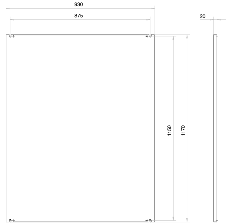
Einbauplatte sendzimirverzinkt
