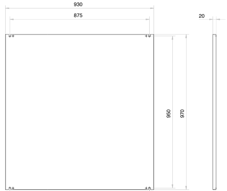
Einbauplatte sendzimirverzinkt
